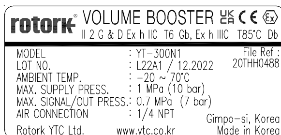
Fig. L-1: YT-300 (UKEX, ATEX)
