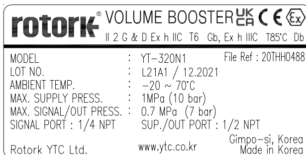
Fig. L-7: YT-320 (UKEX,ATEX)
