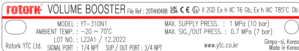
Fig. L-5: YT-310 / 315 (UKEX,ATEX)
