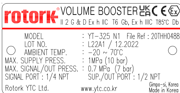
Fig. L-9: YT-325 (UKEX,ATEX)
